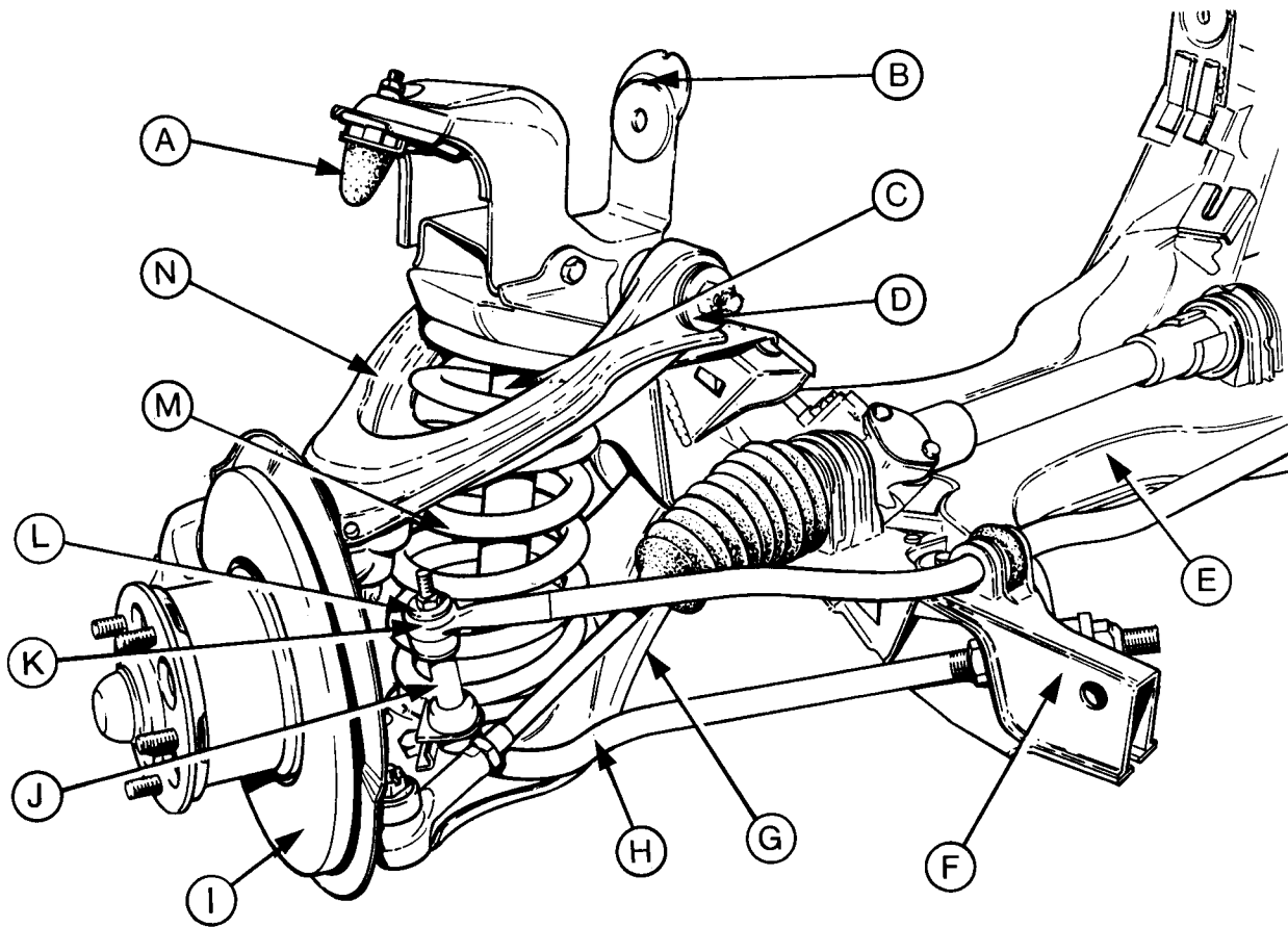
Bild 227 Ansicht der zusammengebauten Vorderradaufhängung.
