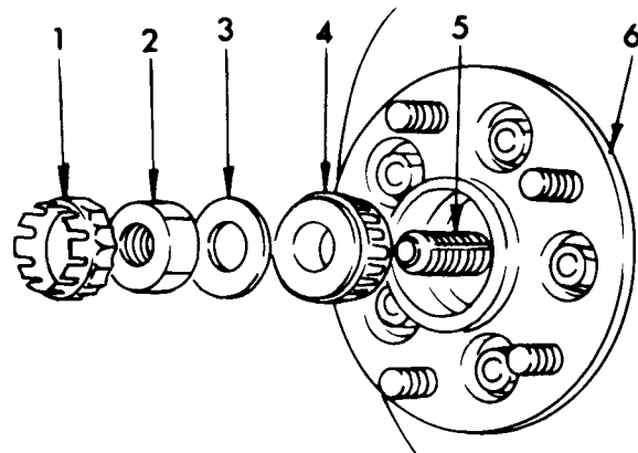
Bild 228 Ansicht der Radlagerteile an der Aussenseite der Radnabe.
