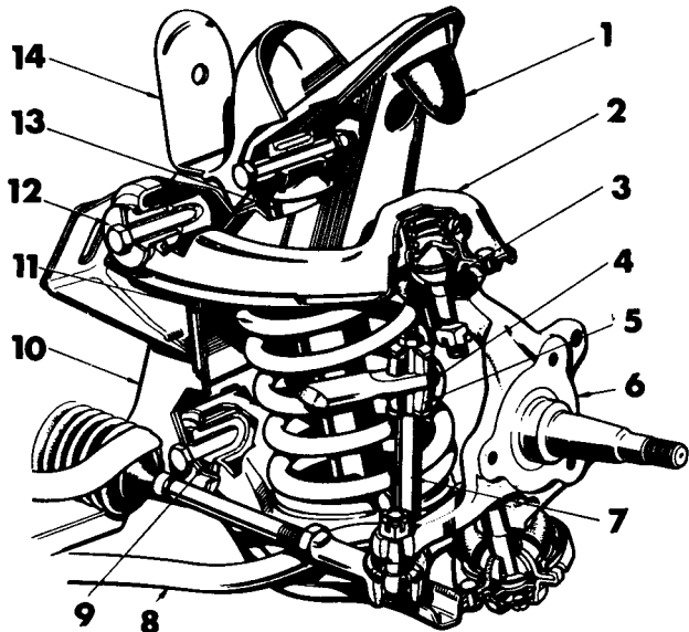
Bild 111 Montagbild der Vorderradaufhängung (eine Seite).
