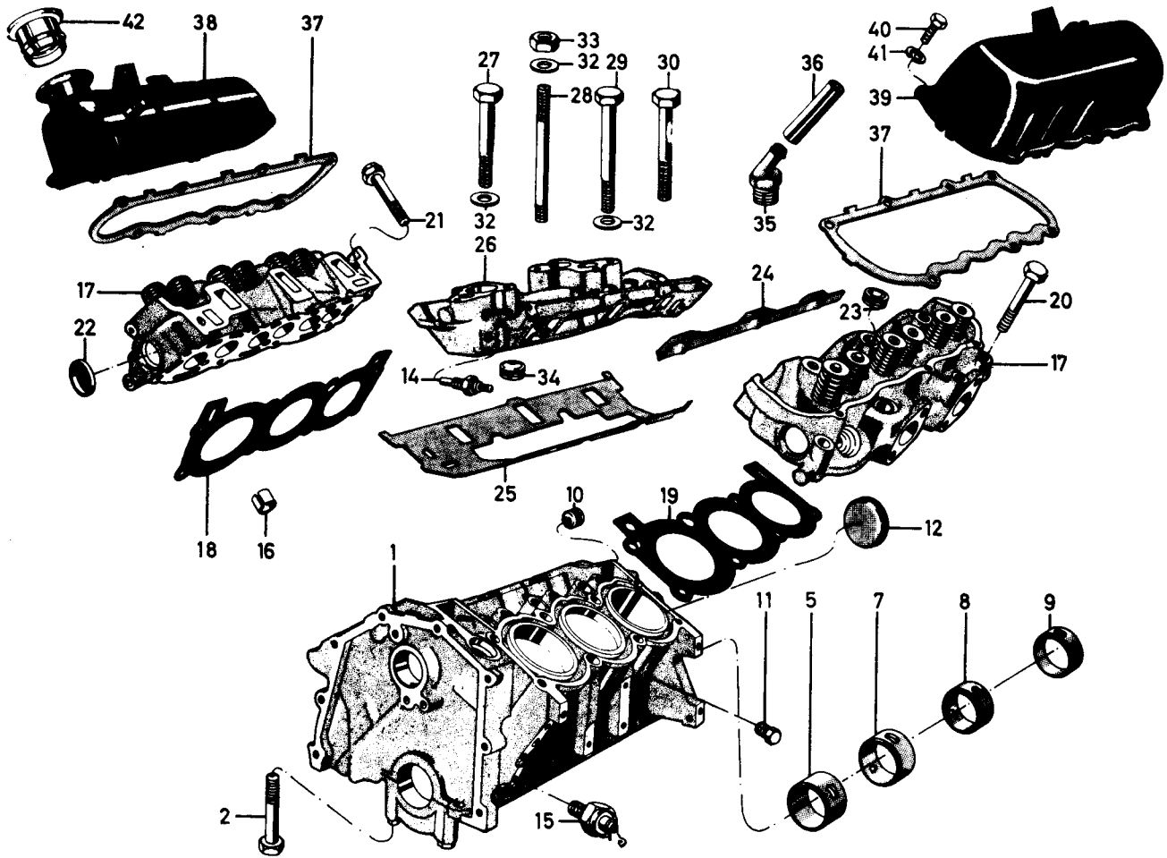
Bild 24 Montagebild von Zylinderblock und Zylinderkopf eines V6-Motors.
