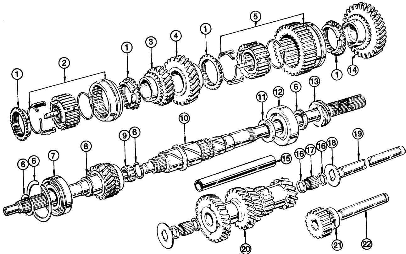
Bild 92 Montagebild der Gangräder und Wellen beim Getriebetyp «B».
