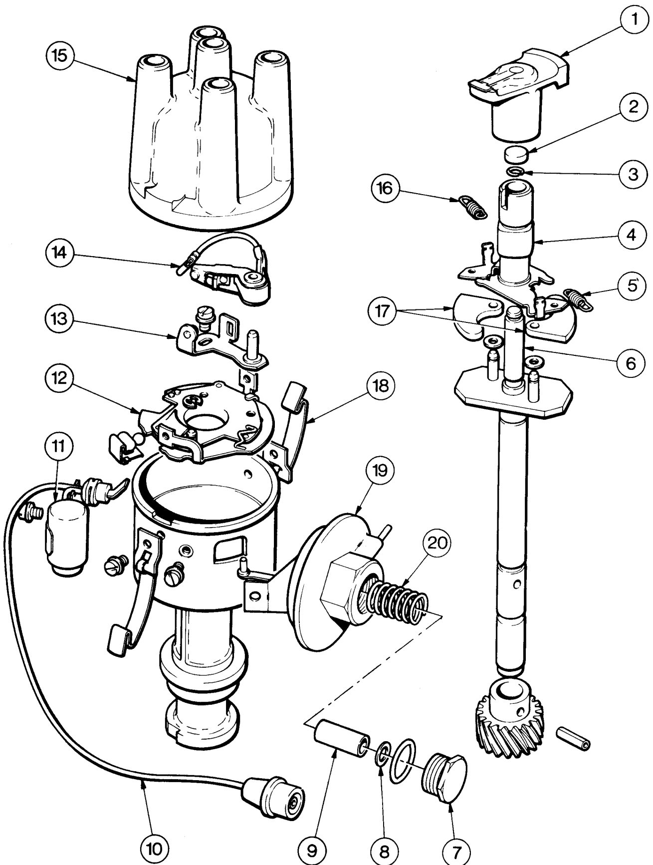
Bild 61 Montagebild eines typischen Bosch-Zündverteilers.
